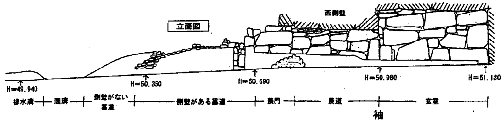
後円部横穴式石室 側壁がある墓道 平面図
