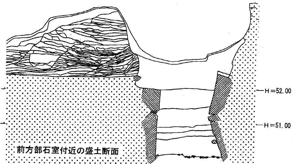
二子塚古墳の墳丘断面図 (1:60)
