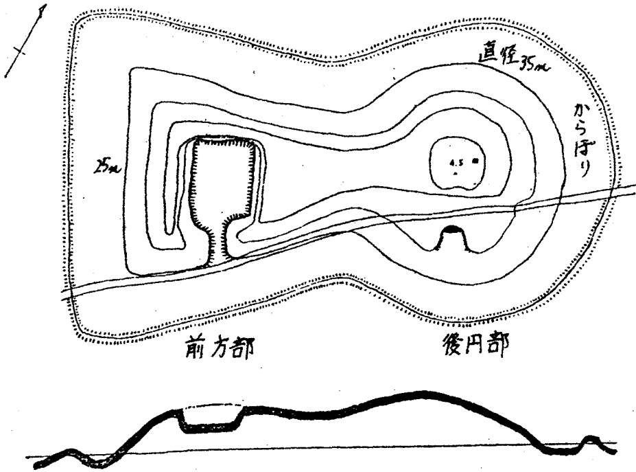
第35図 二子塚古墳実測図 縮尺 1/600
