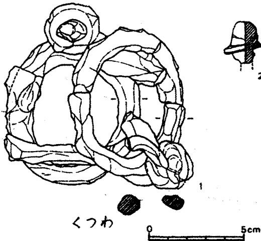
第2図 出土 罎・鉄状金具実測図
