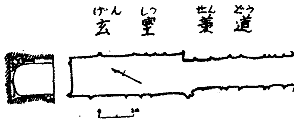
第36図 二子塚古墳石室実測図
