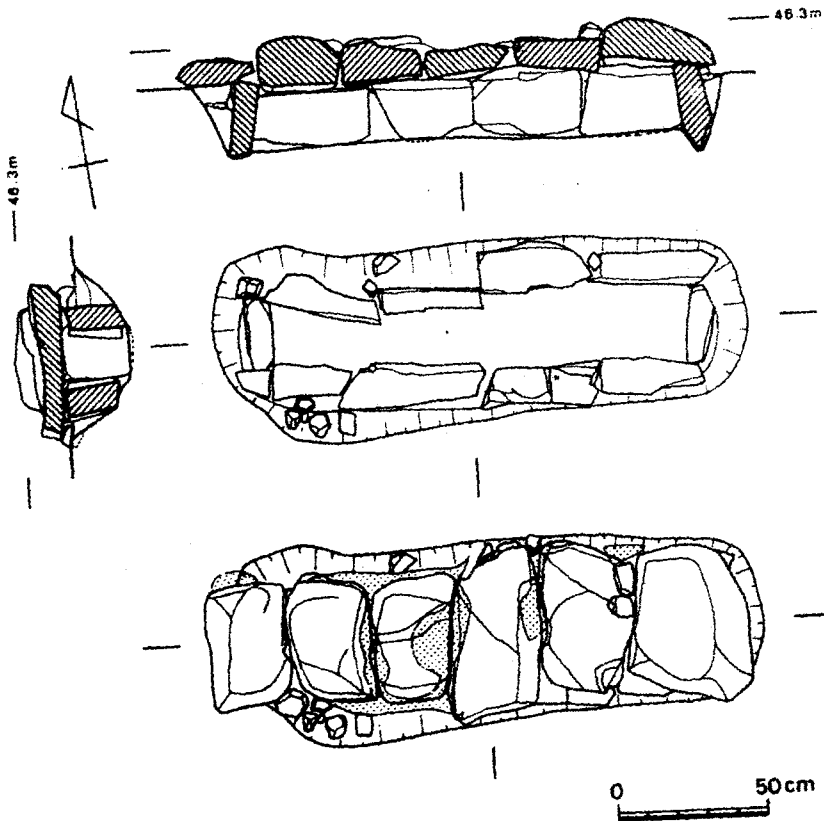
IV-129 稔松古墳石室実測図
