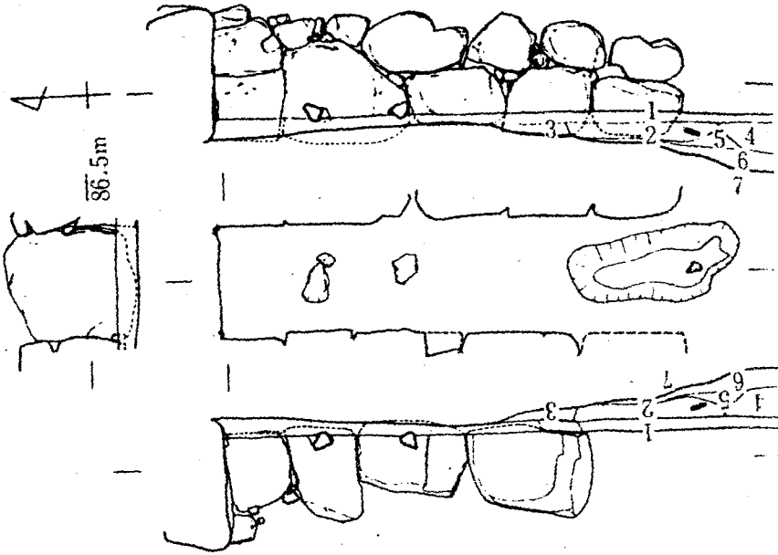
IV-129 稔松古墳石室実測図
