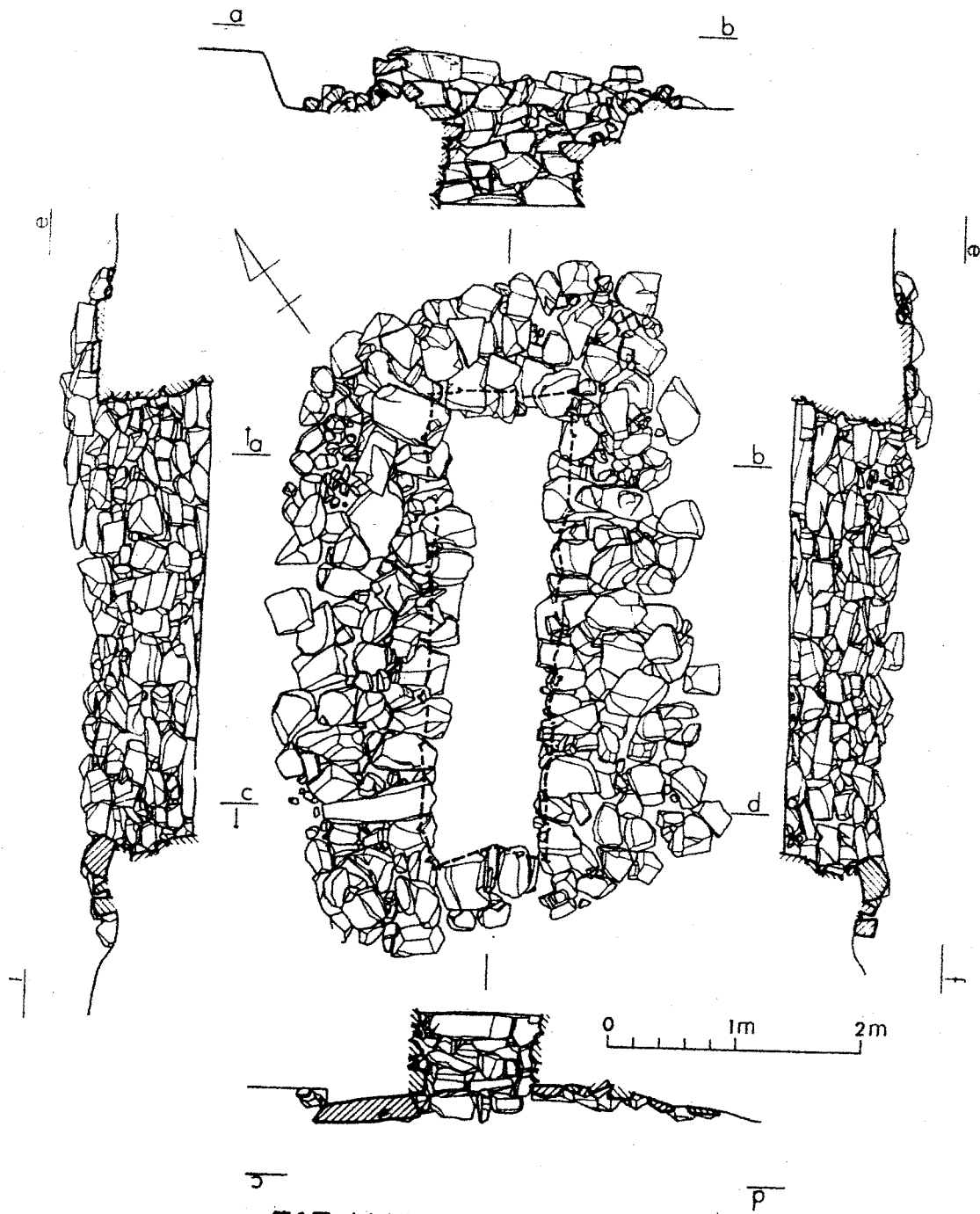
第3图 中小田第1号古墳整穴式石室実測図
