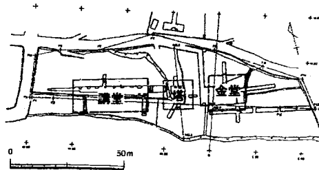
小山池廃寺伽藍配置 (1/2,000)
