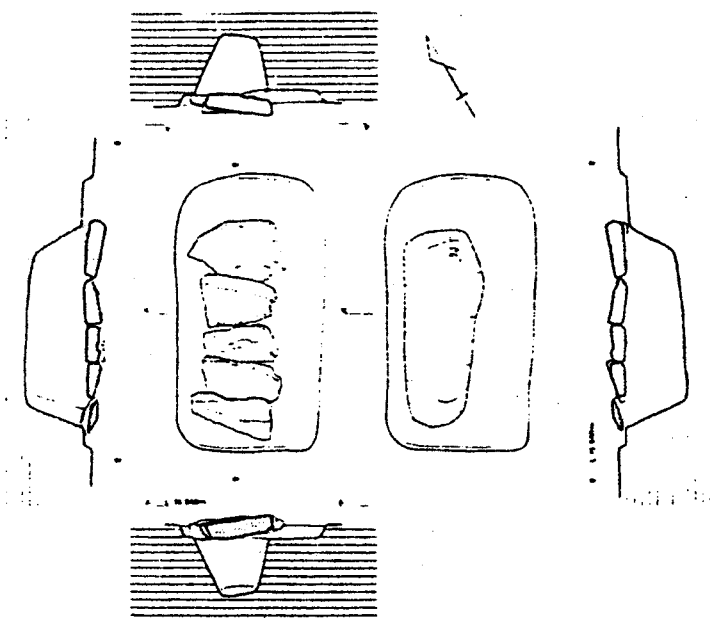
Fig. 67 吹越第8号古墳第2号主体部发掘图
