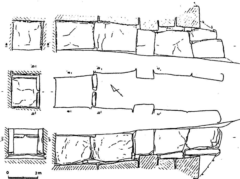
第19圖 大坊古墳石室実測圖
