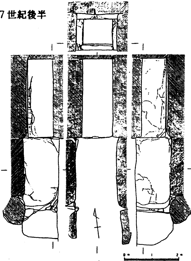
猪の子1号古墳石槨実測図（『装幀』第2集より）
