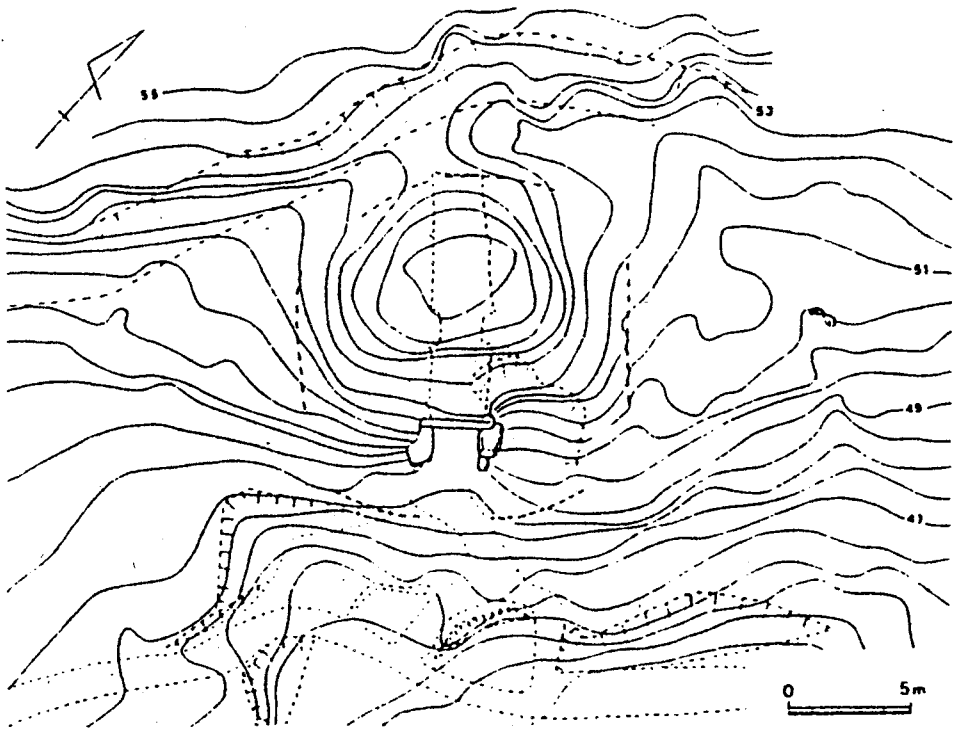
第18圖 大坊古墳墳丘測量圖
