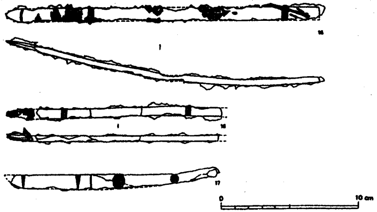
Fig. 12 石鐘山第1号古墳第1号主体部出土遺物実測図
