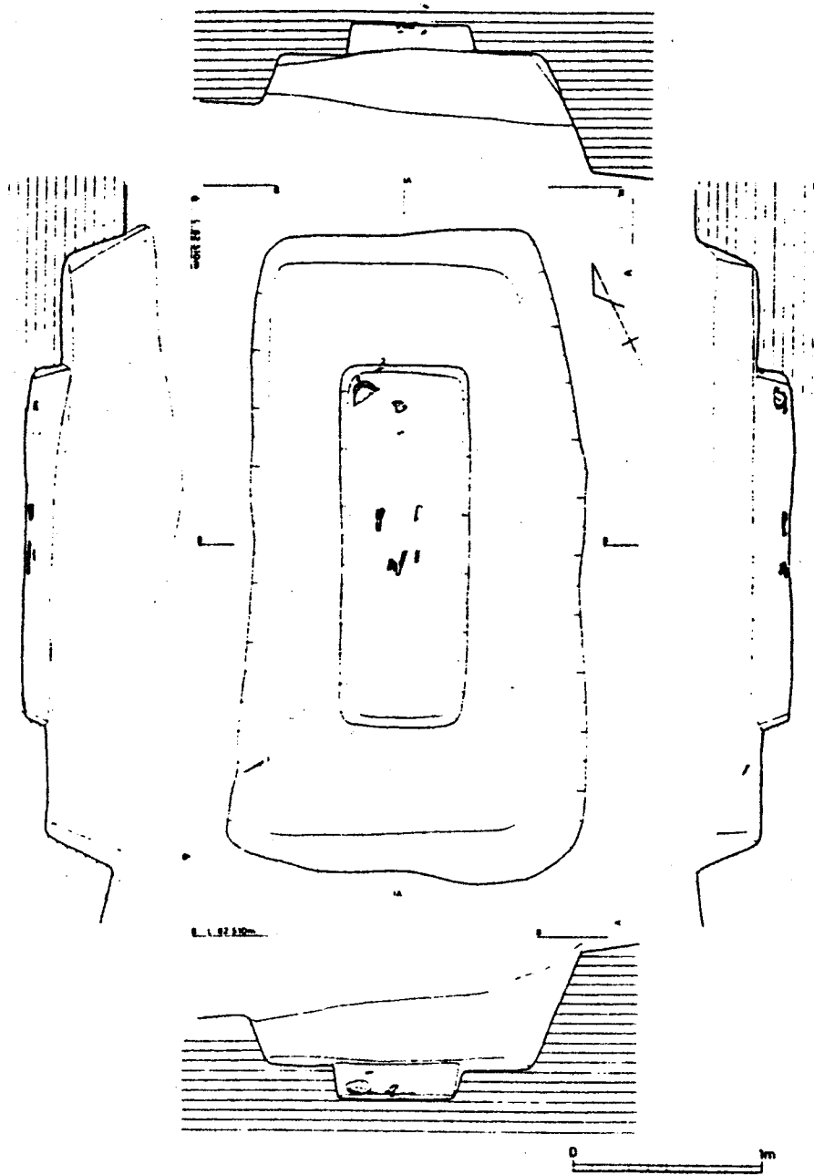
Fig. 22 石鐘山第2号古墳第1号主体部実測図
